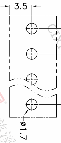
P.C.B.LAYOUT
